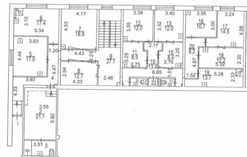
План БТИ
